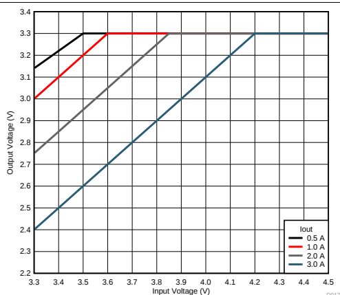
图 20. Voltage Dropout
