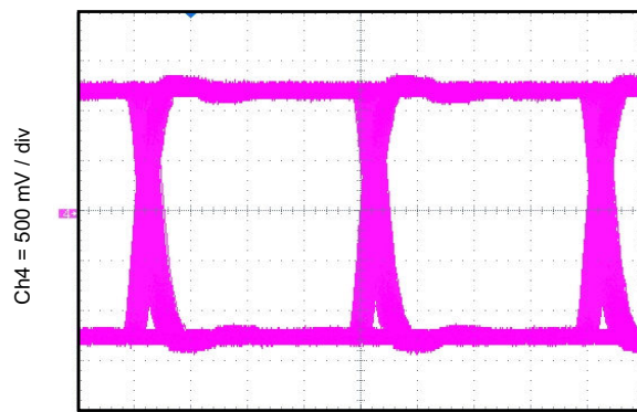
图 8-5. 眼图：100Mbps PRBS 2^{16} - 1 , 2.5 V, 25°C
