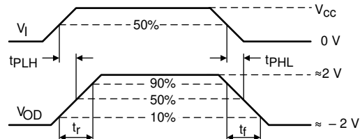
图 7-3. 驱动差分输出上升和下降次数以及传播延迟的测量
