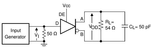
图 7-3. 驱动差分输出上升和下降次数以及传播延迟的测量
