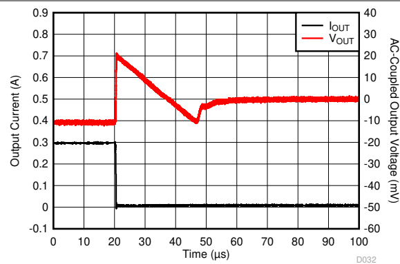
图 5-52. Load Transient
