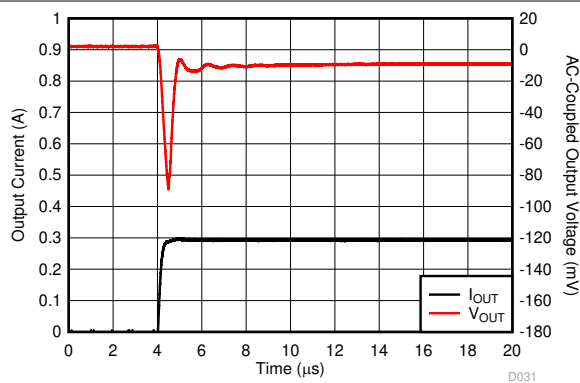
图 5-51. Load Transient
