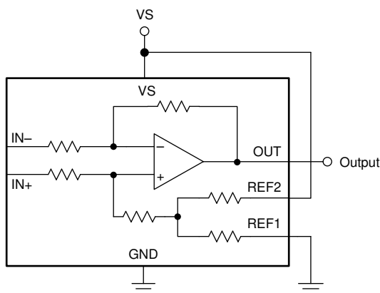
图 8-6. 1/2V_s 电压输出
