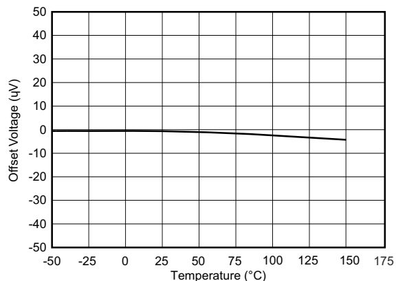
图 7-2. 失调电压与温度间的关系
