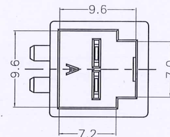
线路板插孔图
