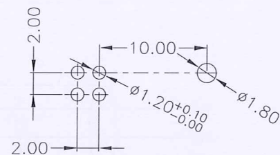
线路板正面插孔图 公差: \pm 0.05
