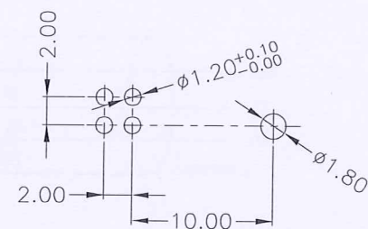
线路板正面插孔图 公差: \pm 0.05
