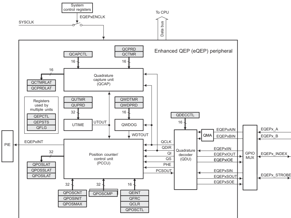
图 7-62. eQEP 方框图
