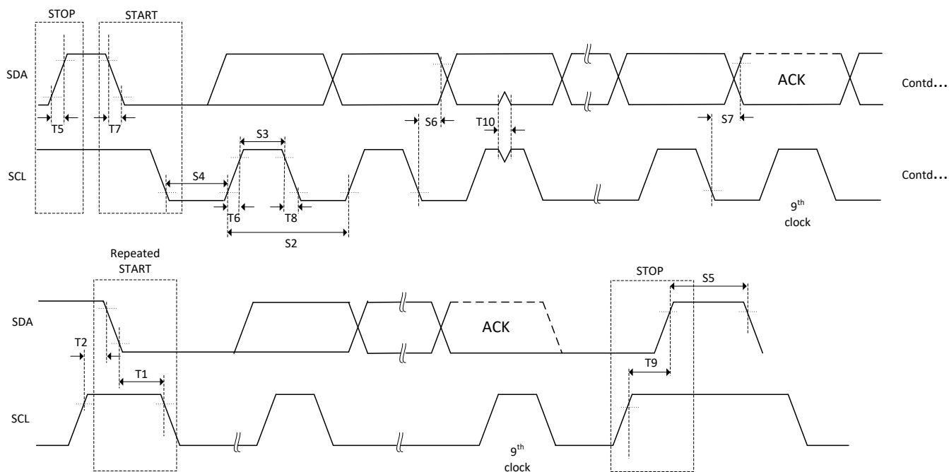
图 7-105. CM-I2C 时序图
