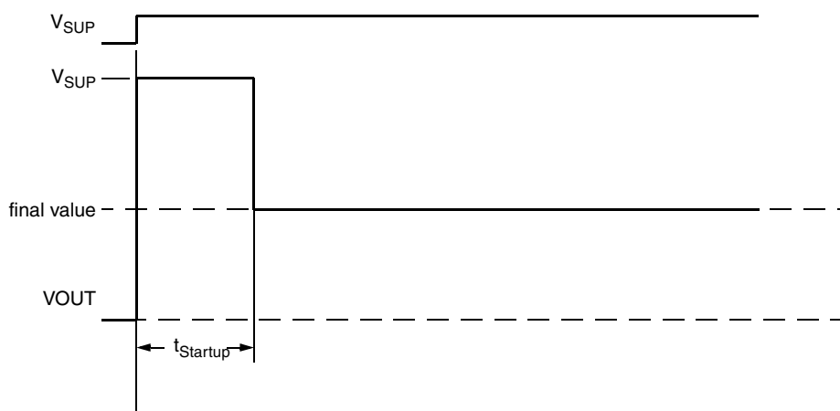
Fig. 4–3: POR timing
