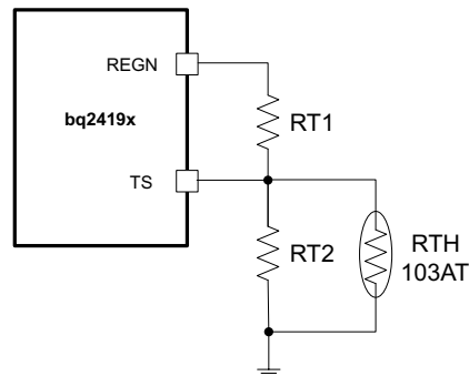
图 15. TS Resistor Network
