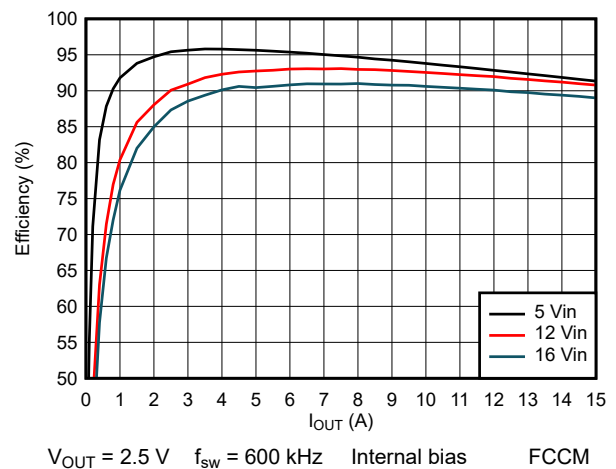
图 8-7. Efficiency
