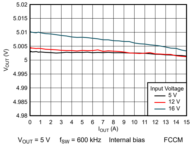
图 8-18. Load Regulation
