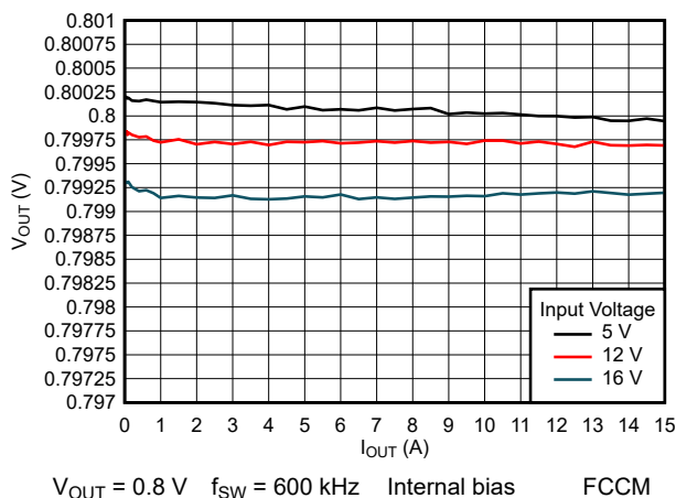
图 8-12. Load Regulation
