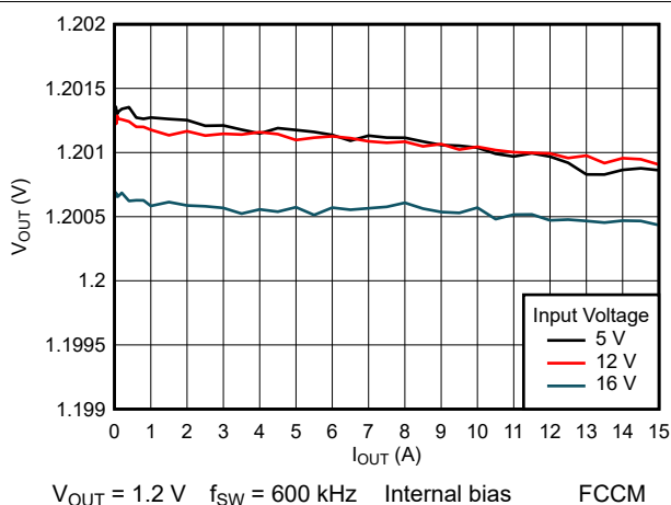
图 8-14. Load Regulation
