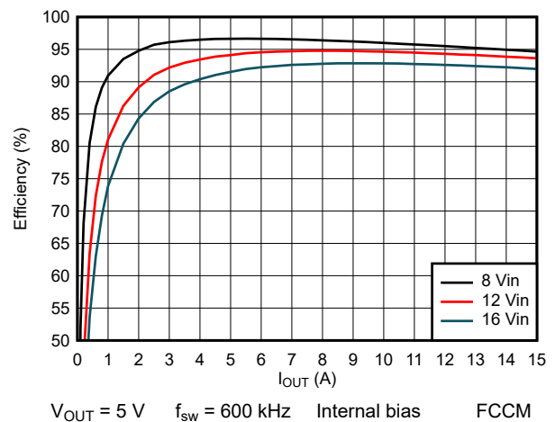
图 8-9. Efficiency
