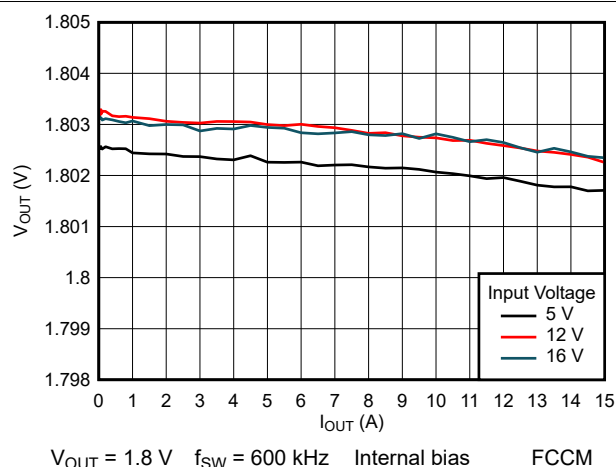
图 8-15. Load Regulation
