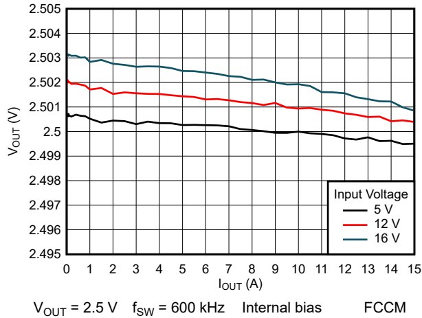
图 8-16. Load Regulation
