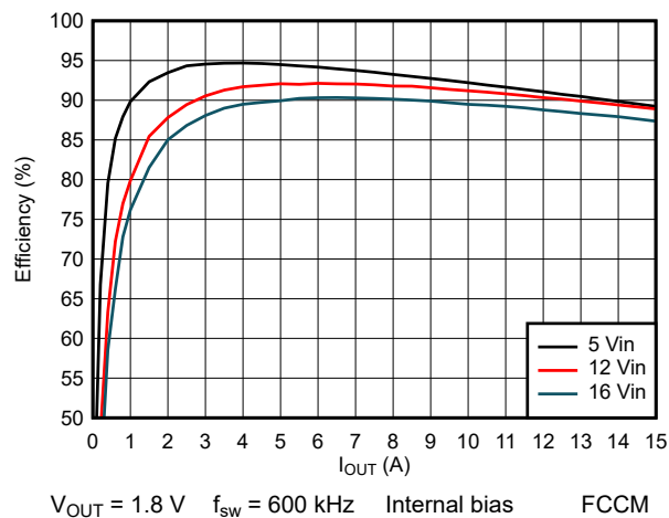
图 8-6. Efficiency
