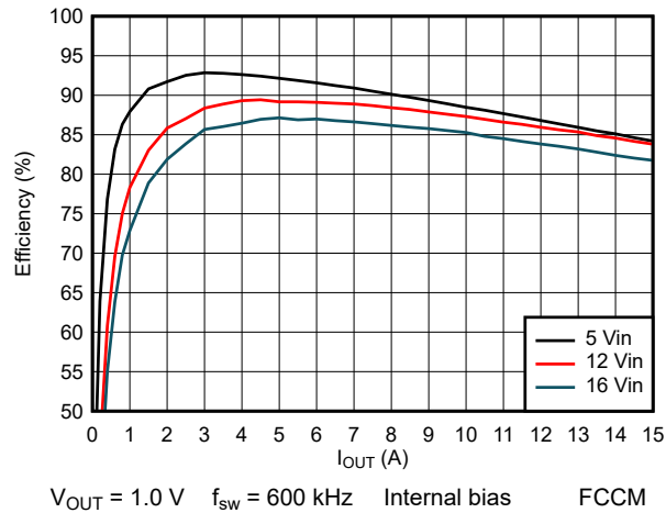
图 8-4. Efficiency
