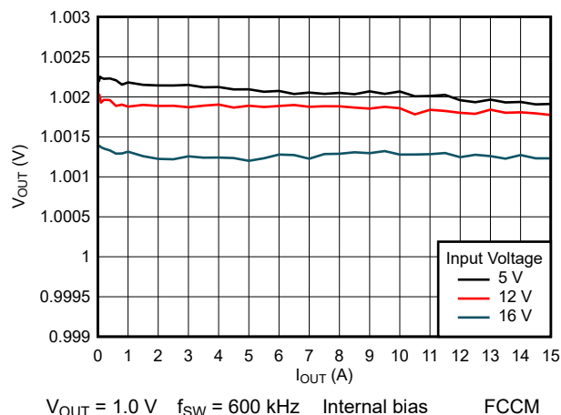
图 8-13. Load Regulation
