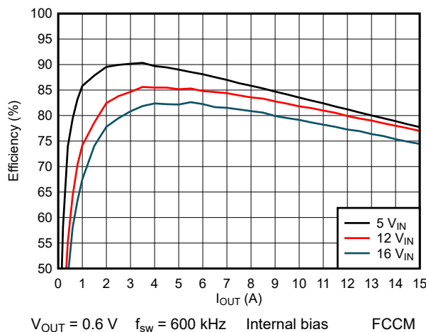
图 8-2. Efficiency
