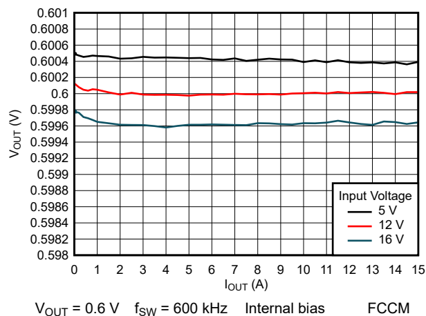
图 8-11. Load Regulation
