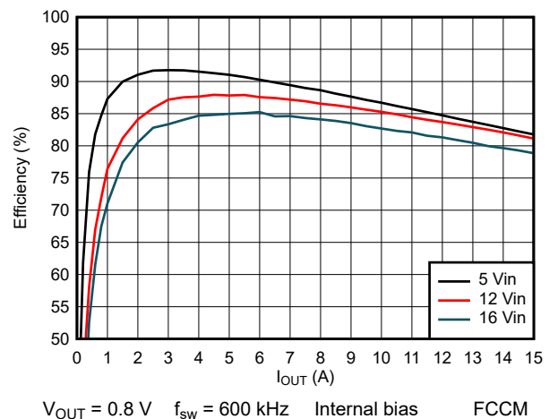
图 8-3. Efficiency
