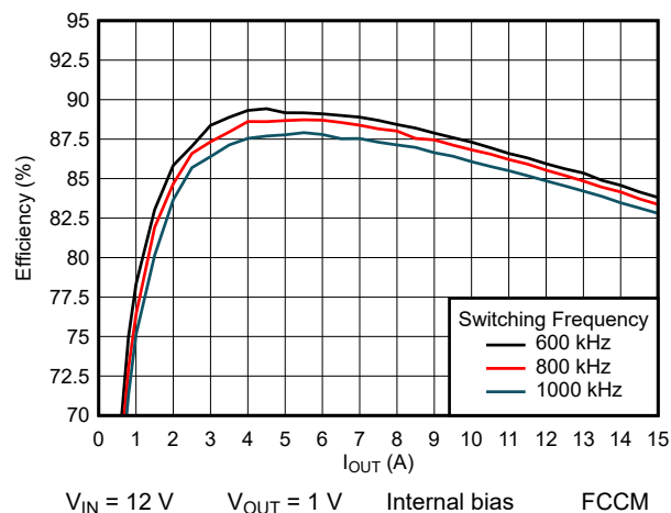
图 8-10. Efficiency
