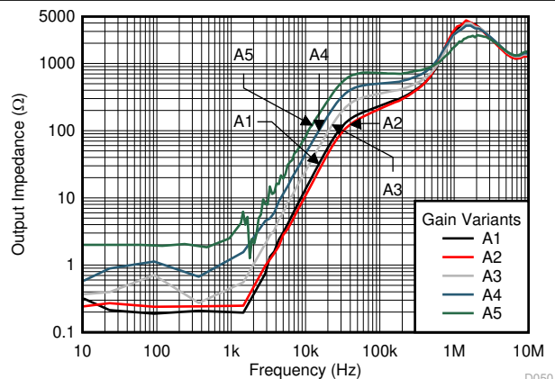
图 6-24. 输出阻抗与频率间的关系
