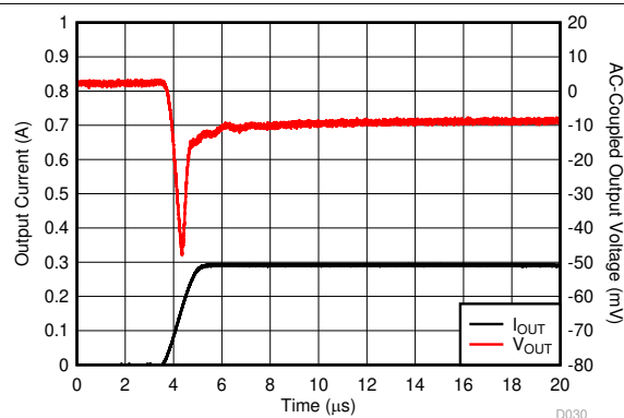
图 5-51. Load Transient
