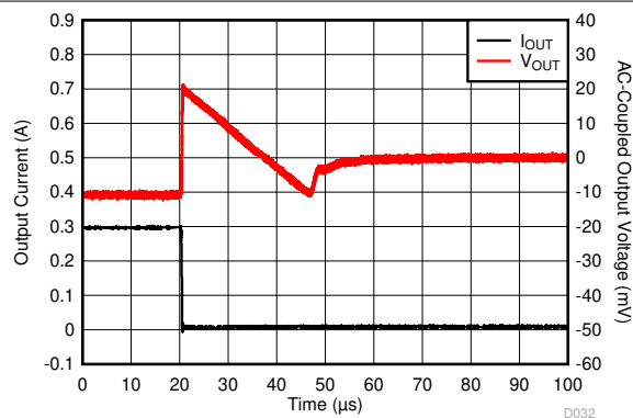
图 5-52. Load Transient
