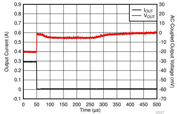
图 5-56. Load Transient
