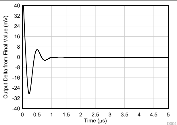
图 7-30. 小信号阶跃响应, G = -1
