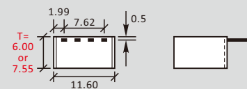
机械尺寸
