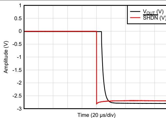
图 7-44. 放大器禁用响应
