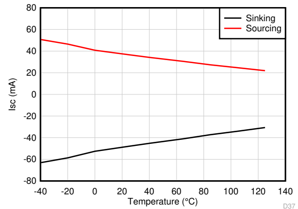
图 7-40. 短路电流与温度间的关系
