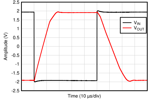
图 7-38. 大信号阶跃响应
