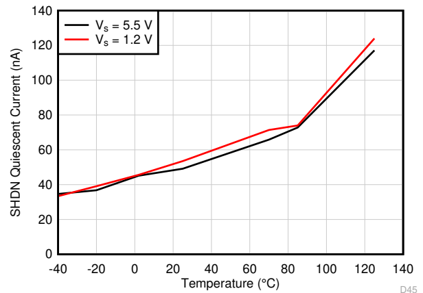
图 7-42. 关断模式静态电流与温度间的关系
