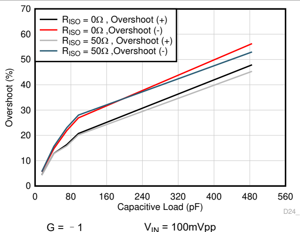
图 7-30. 小信号过冲与容性负载间的关系
