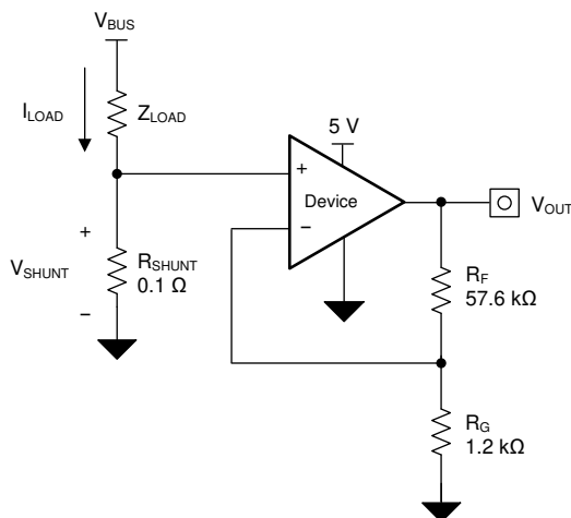
图 9-1. 低侧电流检测应用中的 TLV904x
