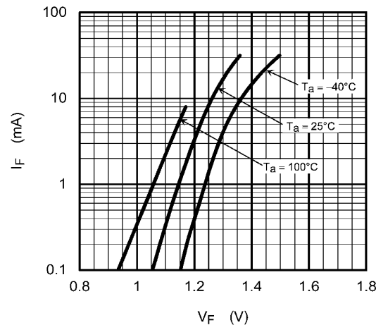
Fig. 12.3 I_F - V_F
