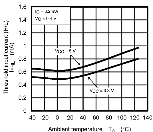
Fig. 12.2.9 I_{FHL} - T_a
