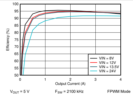
图 10-8. LM62440-Q1 Efficiency
