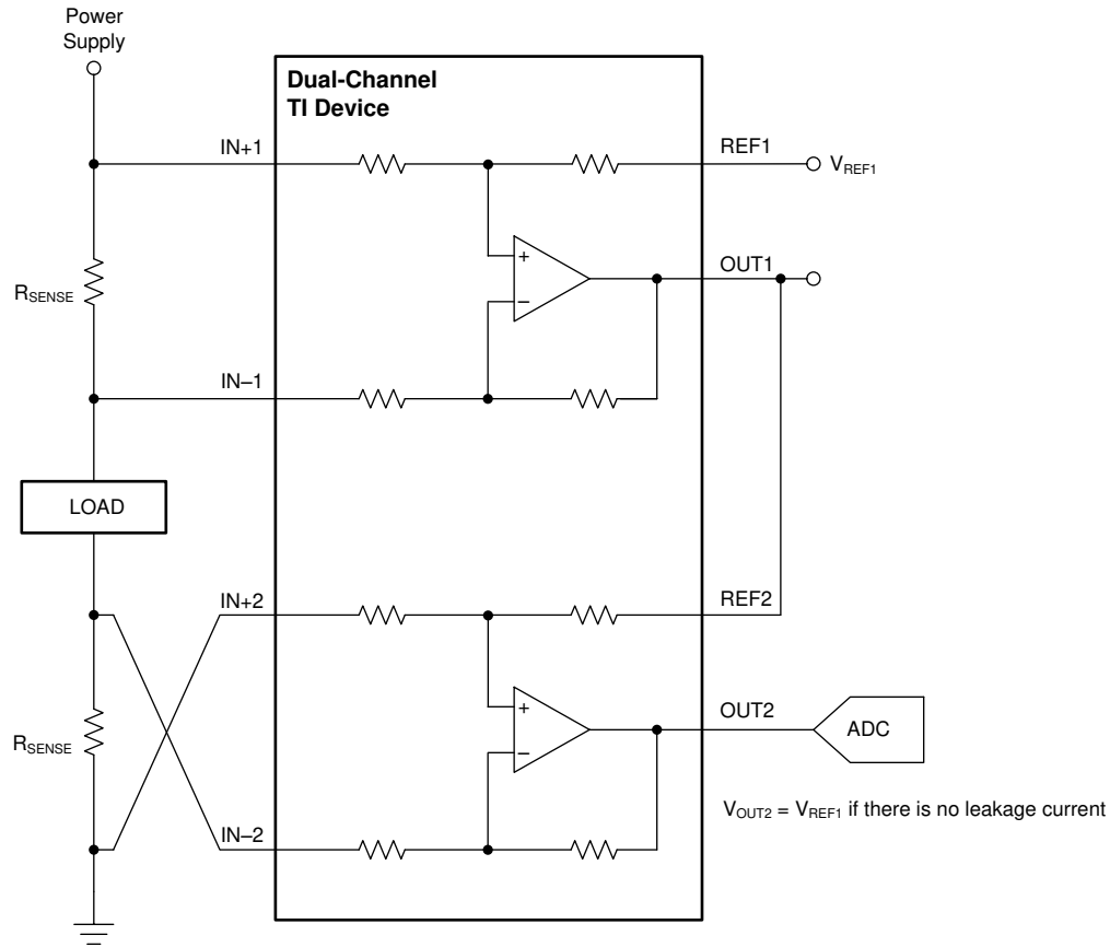
图 8-5. 检测漏电流
