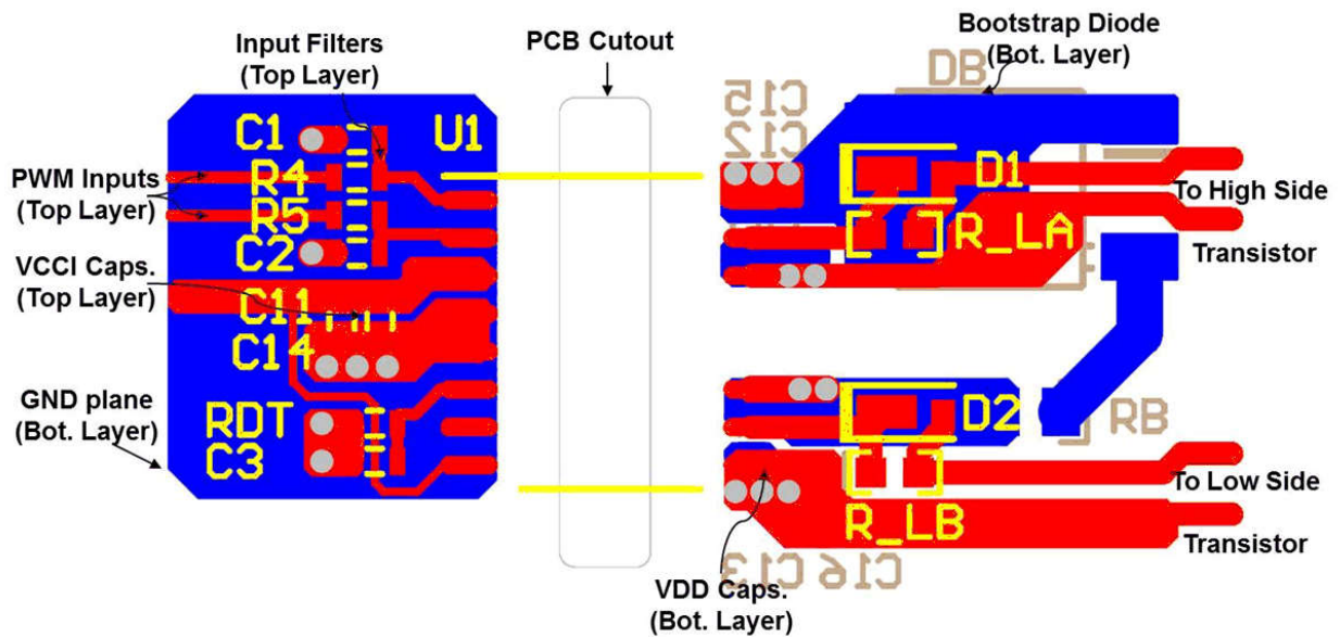
图 11-1. 布局示例
