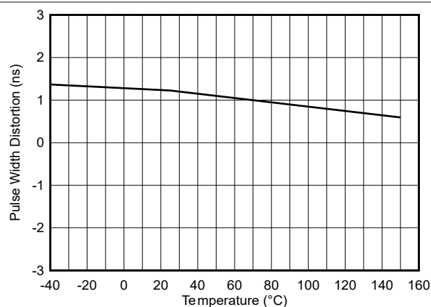
图 6-16. 脉宽失真度
