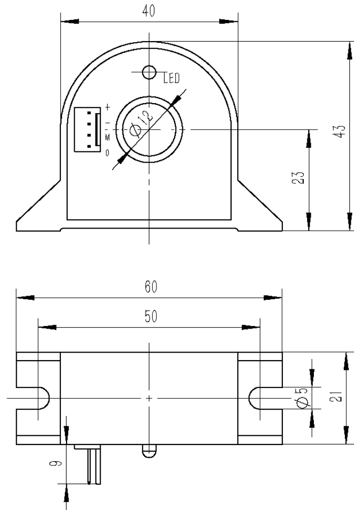
图 1 外形图
