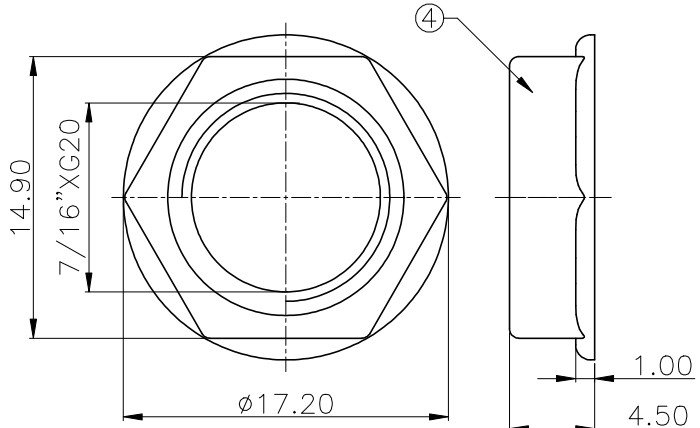
NUT
