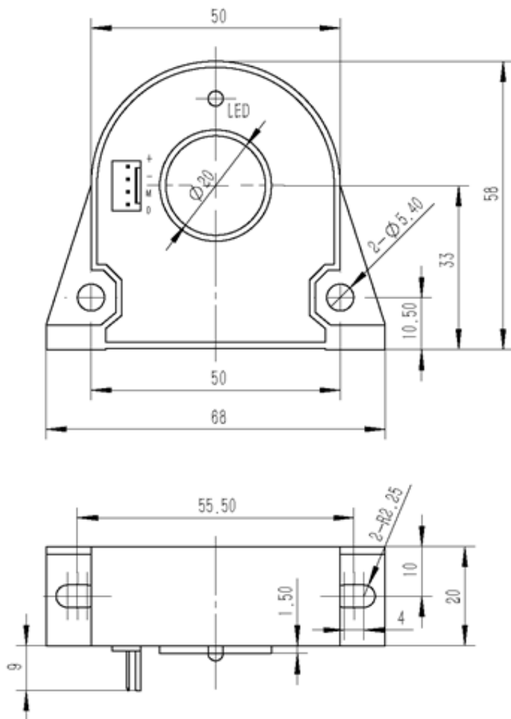
图 1 外形图
