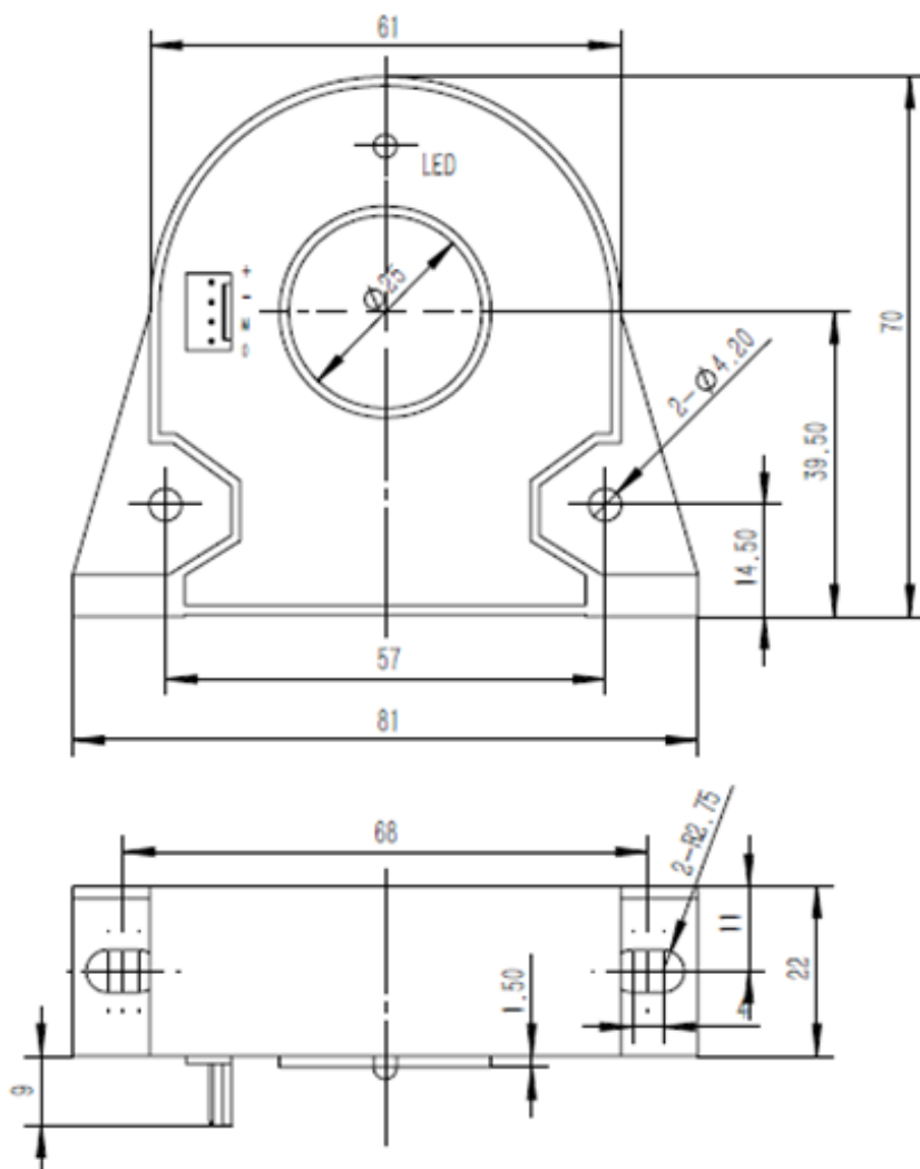
图 1 外形图
