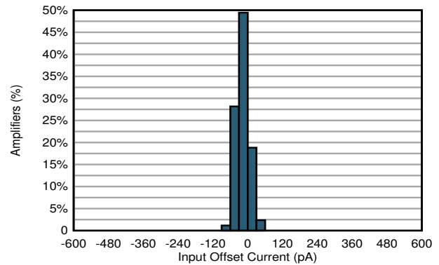
图 7-4. 输入失调电流产生分布
