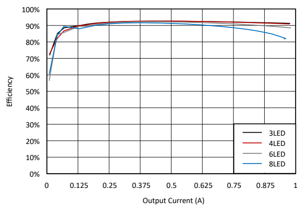
图 6-11. 7\text{ V} 输入电压、 1\text{ A} 输出电流下的效率
