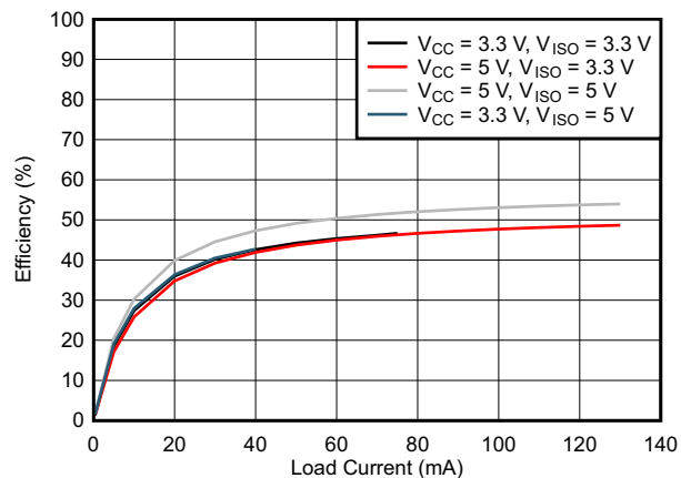
图 7-6. ISOW7841 Efficiency vs Load Current ( I_{ISO} )
