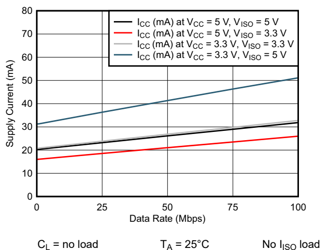
图 7-12. ISOW7841A-Q1 Supply Current vs Data Rate
