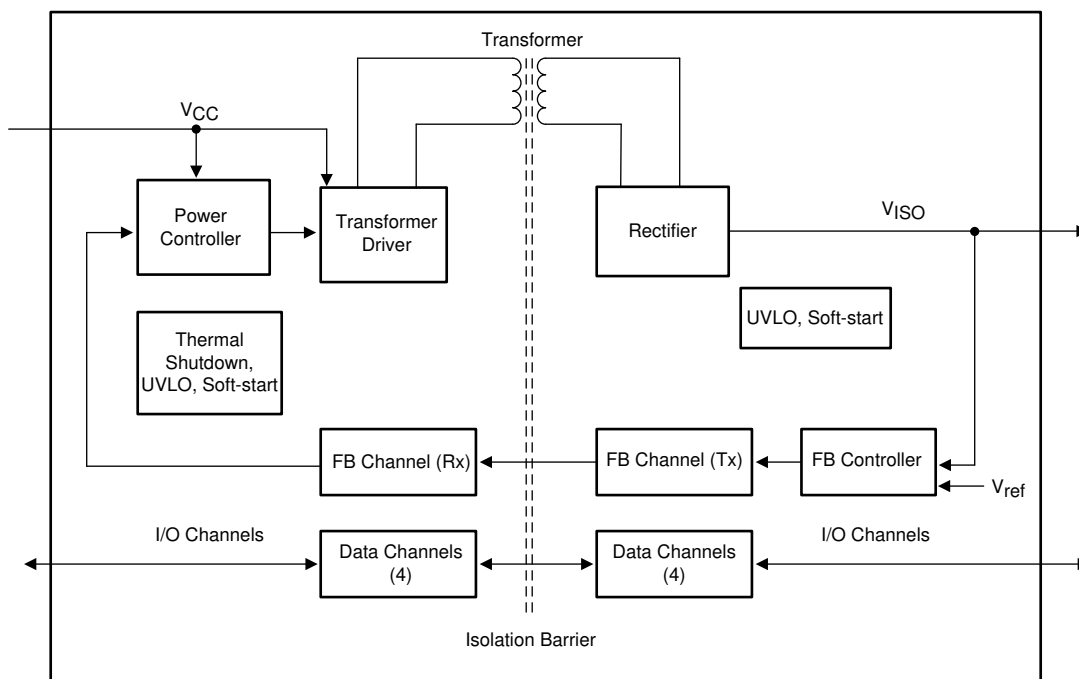
图 9-1. Block Diagram
