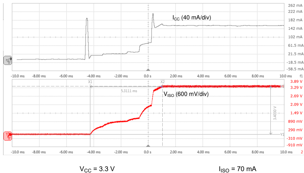
图 10-3. Soft-Start Waveform
