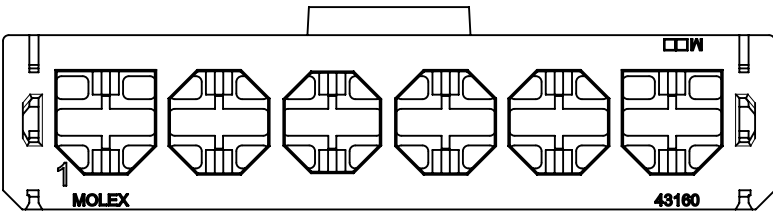
6 CIRCUITS
