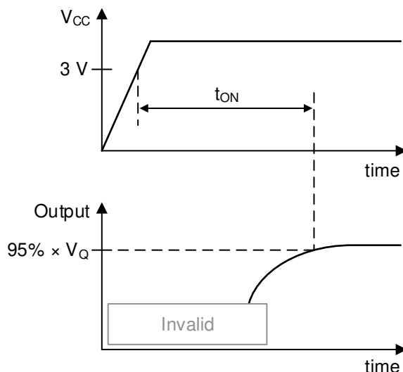
图 6-4. t_{ON} 定义
