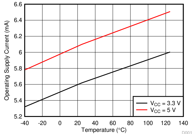
图 5-13. 工作电源电流与温度之间的关系
