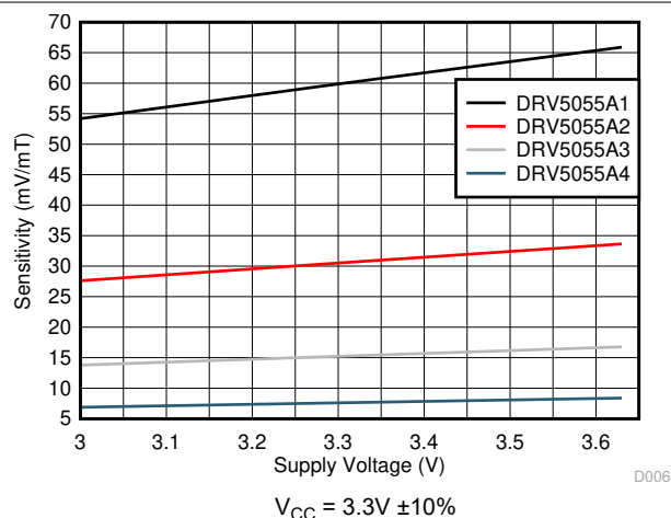
图 5-9. 灵敏度与电源电压之间的关系
