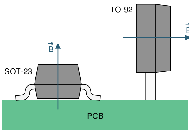
图 6-1. 灵敏度方向
