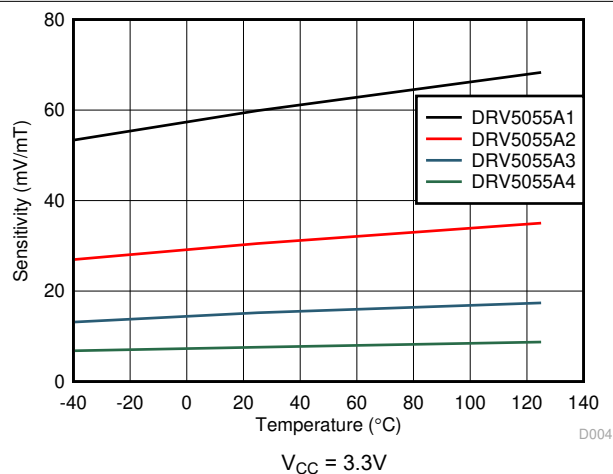
图 5-5. 灵敏度与温度之间的关系
