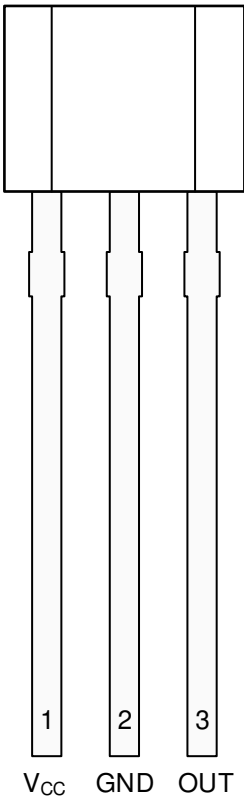
图 4-2. LPG 封装 3 引脚 TO-92 顶视图
