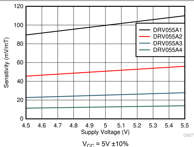
图 5-10. 灵敏度与电源电压之间的关系
