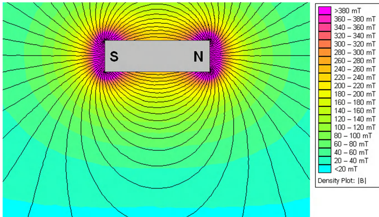
图 7-3. 仿真磁通
