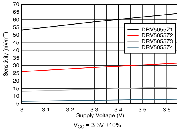
图 5-11. 灵敏度与电源电压之间的关系
