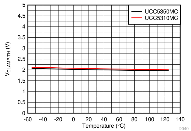
图 6-26. V_{Clamp-TH} vs Temperature
