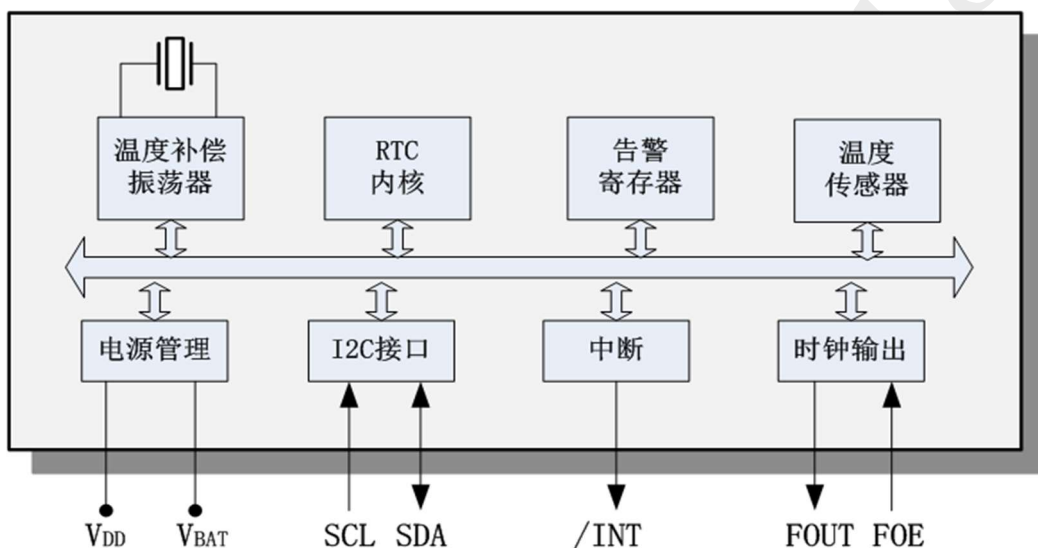
图 1 原理框图
