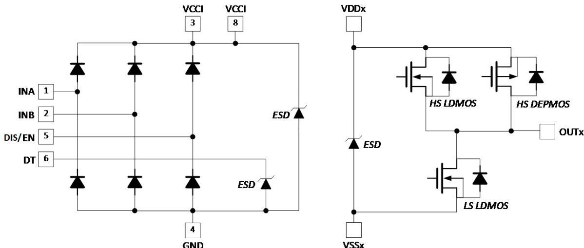
图 8-3. ESD 结构
