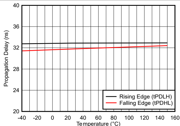
图 6-16. 传播延迟, 上升沿和下降沿
