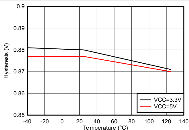
图 6-14. INA/INB/DIS 高和低阈值迟滞
