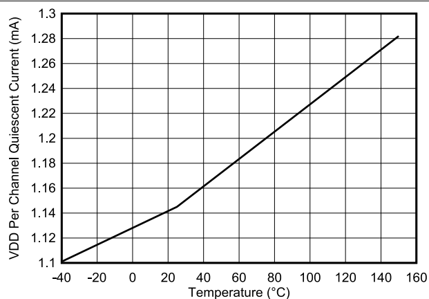
图 6-7. 每通道 VDD 静态电流 ( I_{VDDA} 、 I_{VDDb} )
