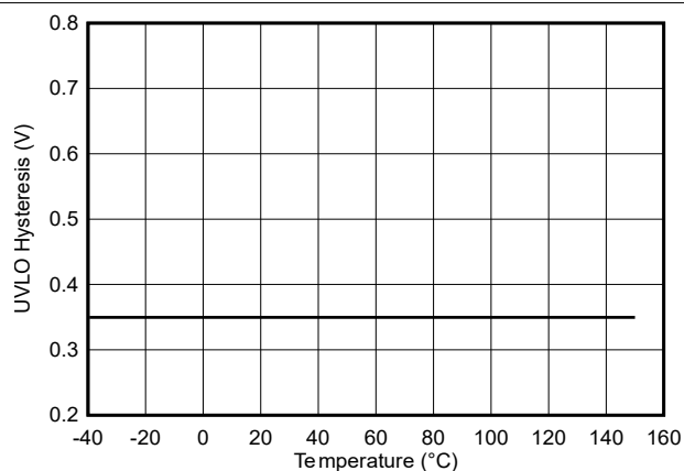
图 6-11. 5V VDD UVLO 迟滞电压
