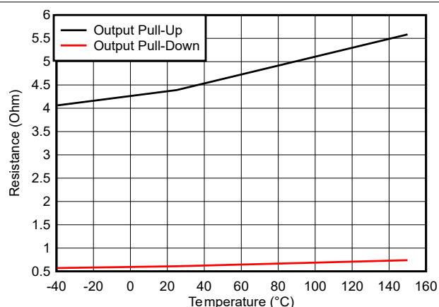
图 6-15. OUT 上拉和下拉电阻
