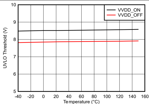
图 6-12. 8V VDD UVLO 阈值电压
