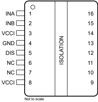
图 5-3. DW 封装 16 引脚 SOIC 顶视图
