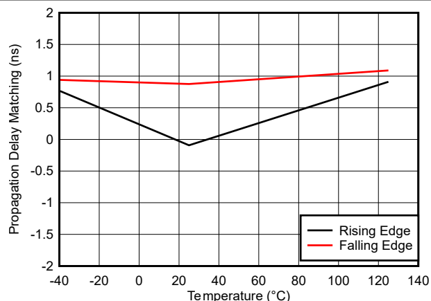
图 6-17. 传播延迟匹配, 上升沿和下降沿
