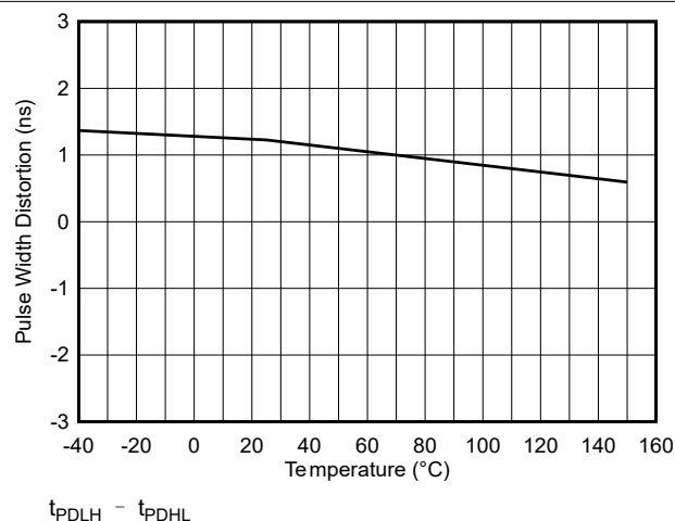
图 6-18. 脉宽失真度
