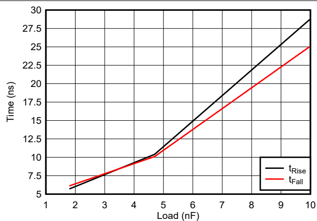
图 6-19. 上升时间和下降时间与负载间的关系
