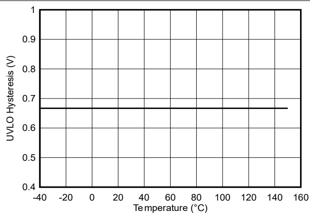
图 6-13. 8V VDD UVLO 阈值迟滞电压
