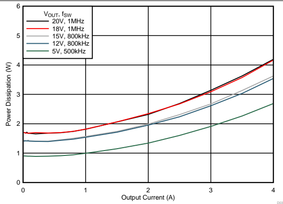
图 27. Power Dissipation
