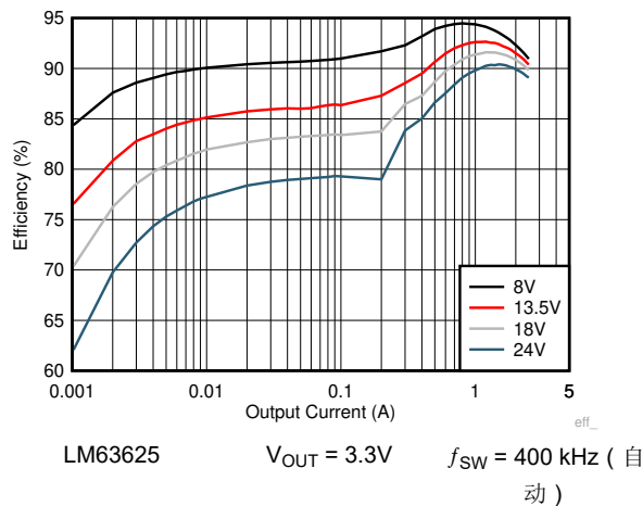
图 8-12. 效率
