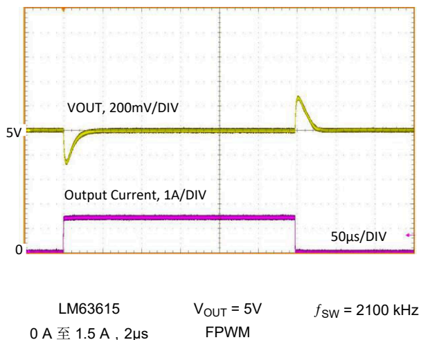
图 8-29. 负载瞬态
