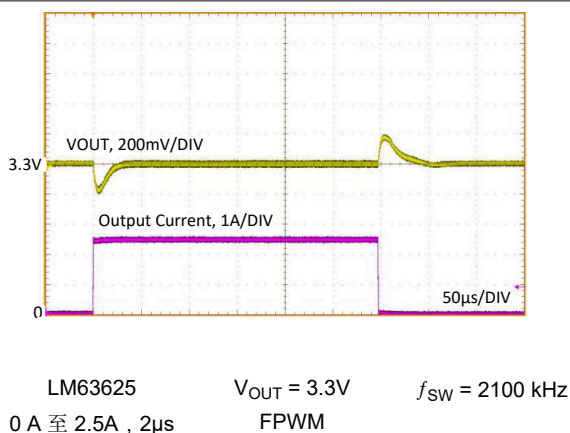
图 8-26. 负载瞬态
