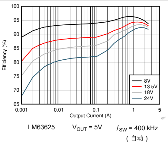
图 8-8. 效率
