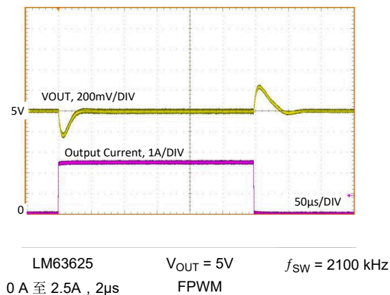
图 8-28. 负载瞬态
