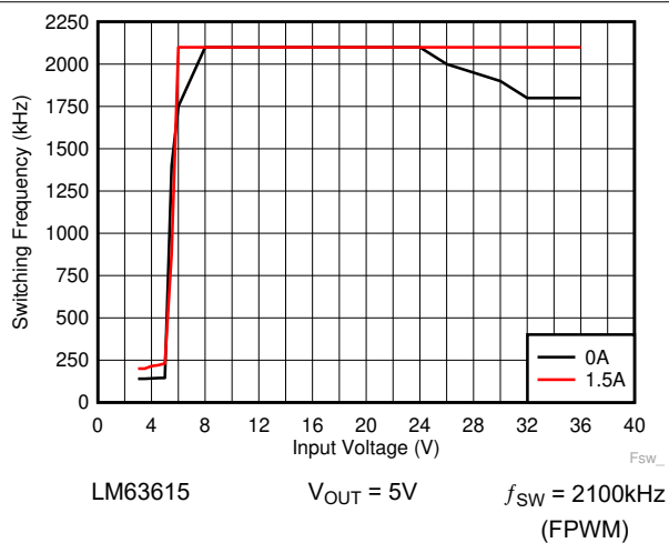
图 8-25. 开关频率与输入电压间的关系
