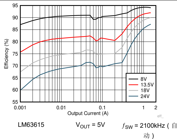
图 8-11. 效率
