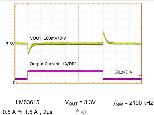
图 8-31. 负载瞬态
