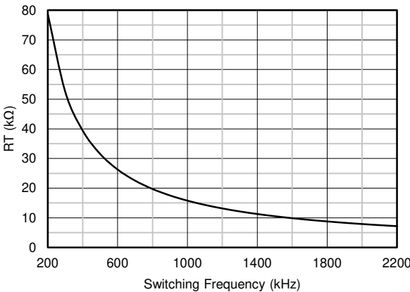
图 7-1. 开关频率与 R_T 间的关系
