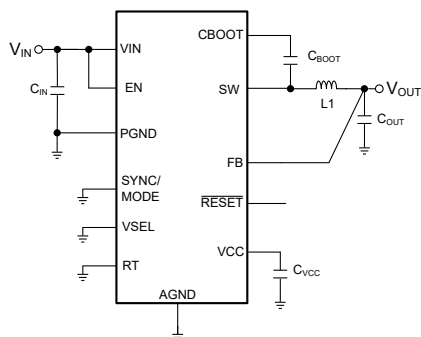
简化原理图
