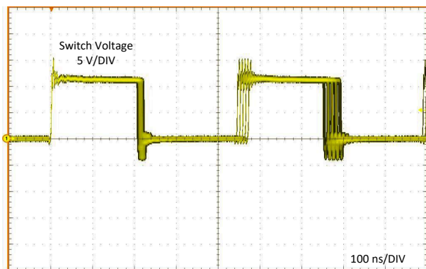
图 7-8. 有展频的典型 PWM 开关波形, V_{IN} = 12V , V_{OUT} = 5V , I_{OUT} = 2.5A , f_{SW} = 2100kHz
