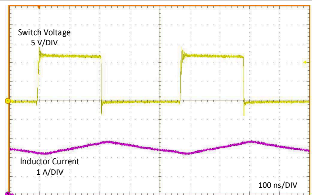
图 7-7. 没有展频的典型 PWM 开关波形， V_{IN} = 12V ， V_{OUT} = 5V ， I_{OUT} = 2.5A ， f_{SW} = 2100kHz
