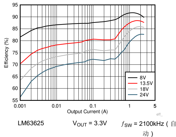
图 8-13. 效率
