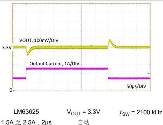
图 8-30. 负载瞬态
