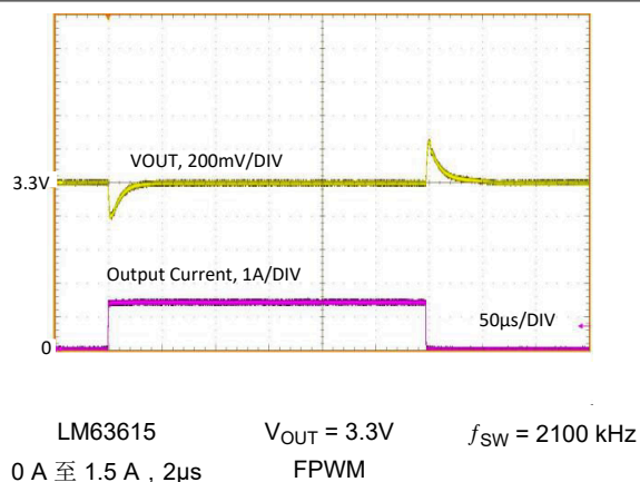
图 8-27. 负载瞬态
