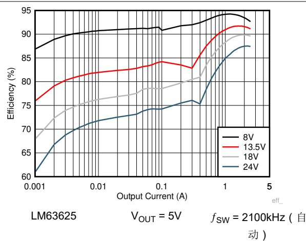
图 8-9. 效率
