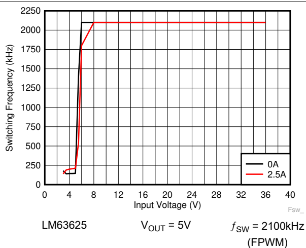
图 8-23. 开关频率与输入电压间的关系
