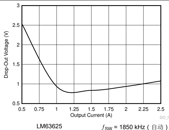
图 8-35. 1.85MHz 时电压降与输出电流间的关系
