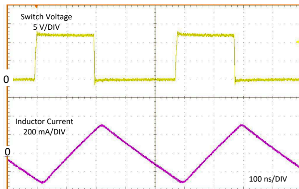
图 7-9. 典型 PWM 开关波形, FPWM, V_{IN} = 12V , V_{OUT} = 5V , I_{OUT} = 0A , f_{SW} = 2100kHz
