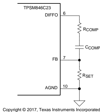
图 15. R_{SET} Resistor
