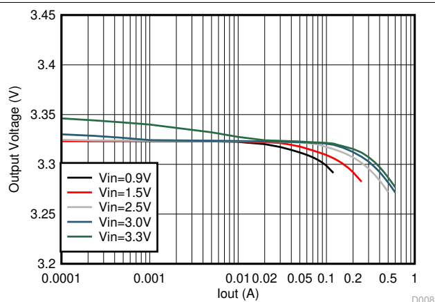
图 6-2. Load Regulation
