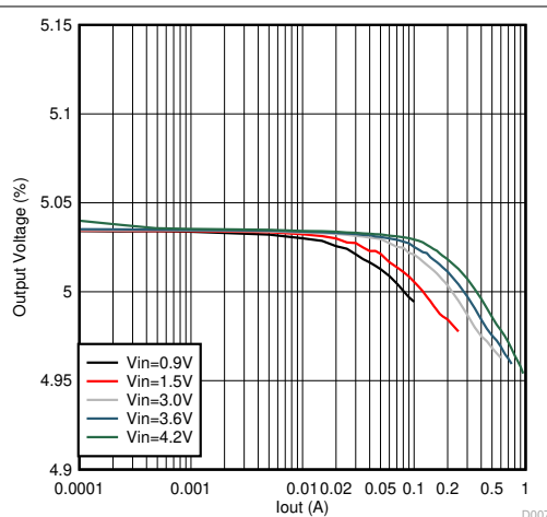
图 6-4. Load Regulation
