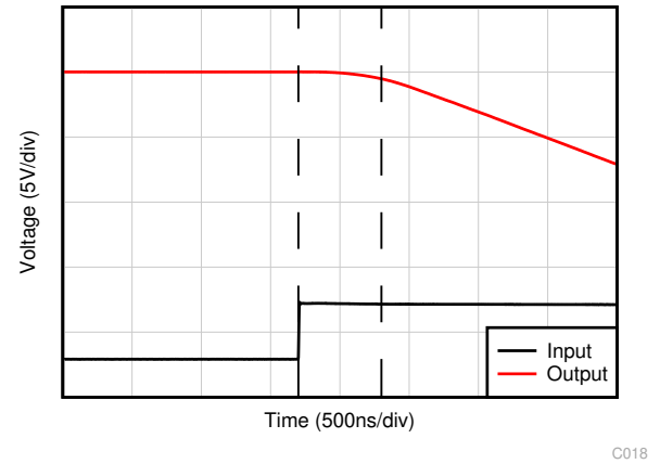
图 6-30. 正过载恢复
