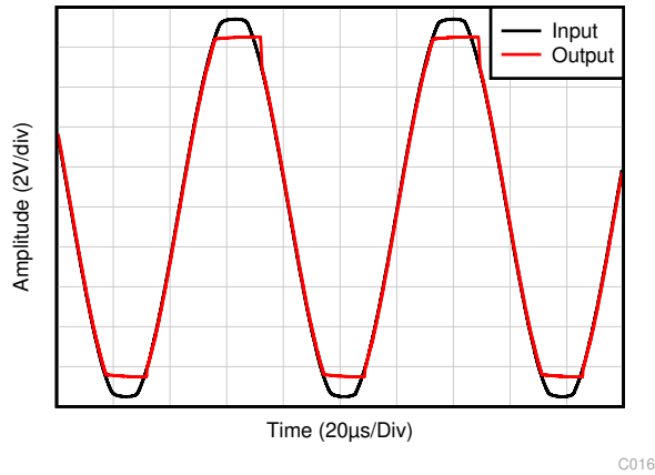
图 6-29. 无相位反转
