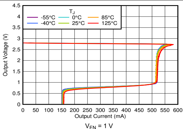
图 5-44. Current Limit
