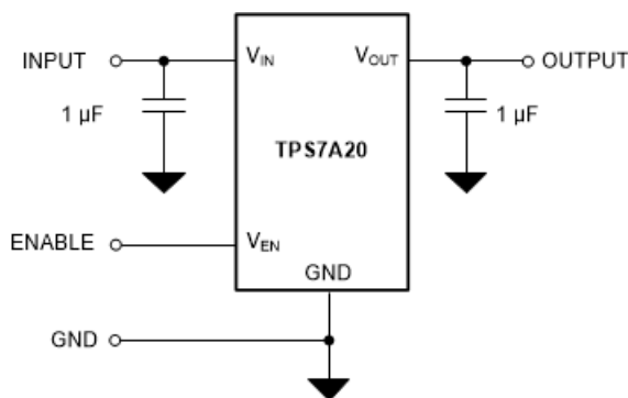
应用原理图
