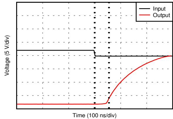
图 6-30. 无相位反转
