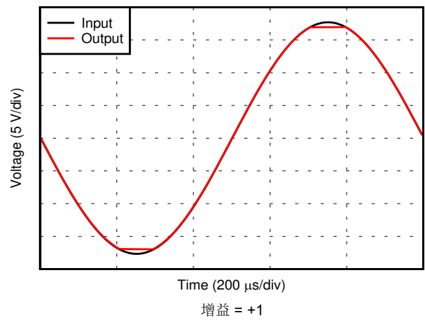
图 6-30. 无相位反转
