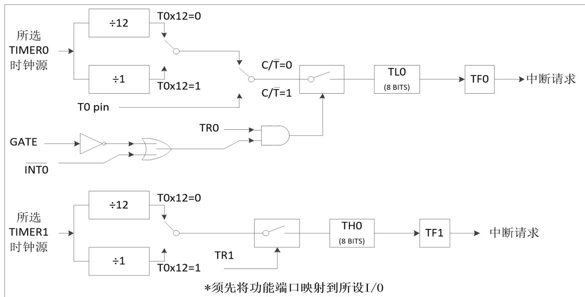
ure 9-4 TIMER0 方式 3 功能框图
