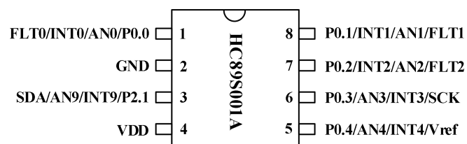
Figure 1-4 SOP8 引脚配置图
