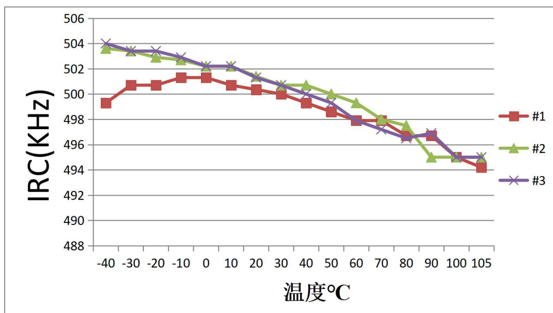
Figure 22-4 内部高频RC32M/500-温度特性曲线图
