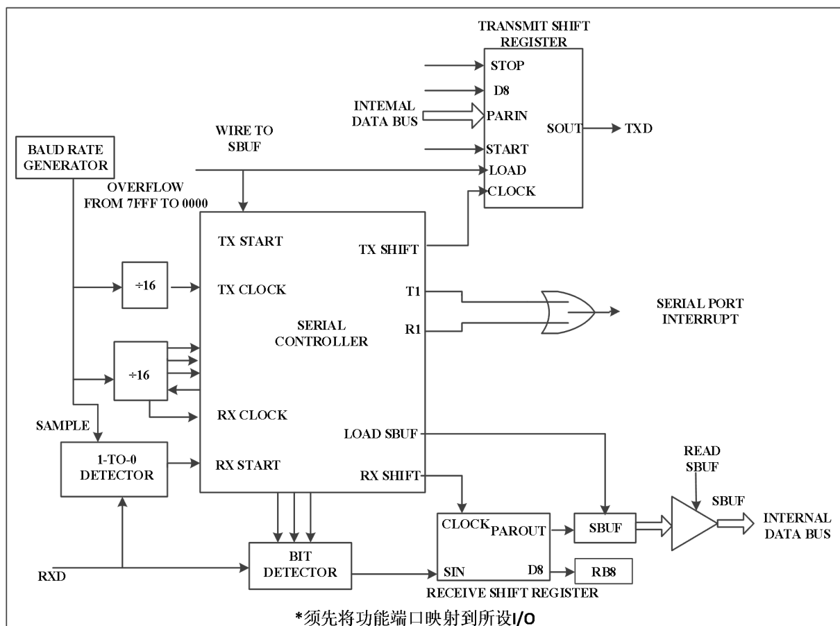
Figure 13-10 UART 模式 3 功能框图
