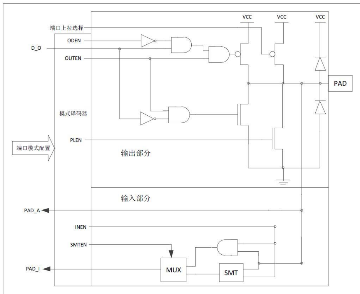
Figure 7-1 I/O 功能框图
