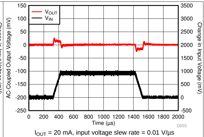
图 20. V_{IN} Transient
