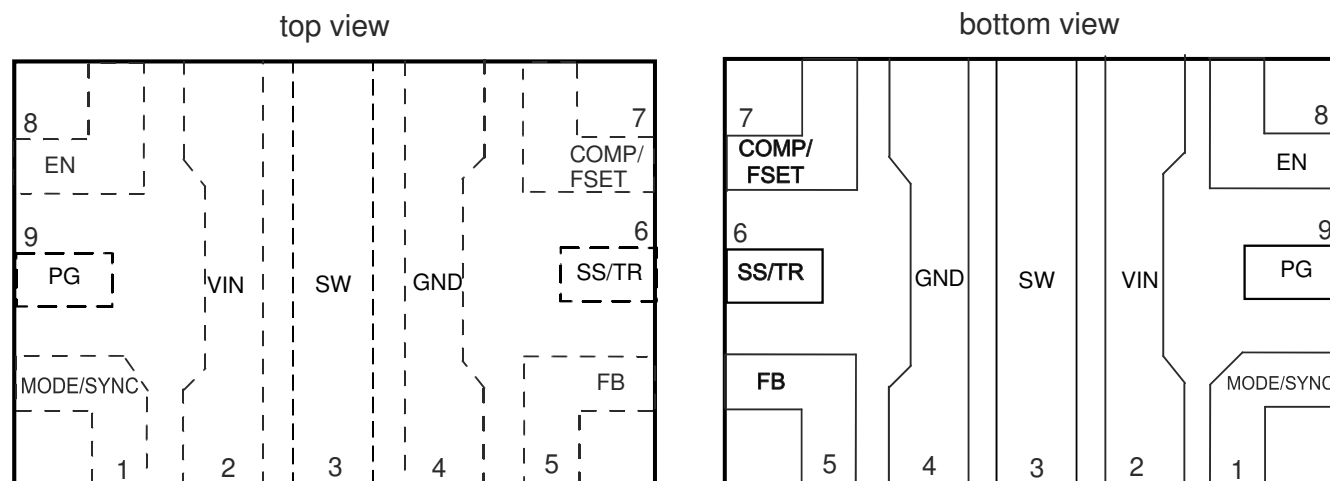
图 6-1. RWY Package 9 Pin (VQFN)
