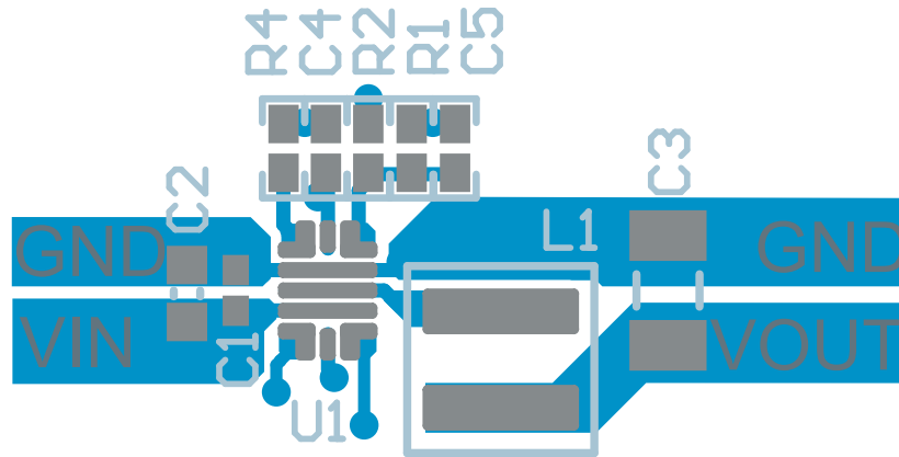
图 10-63. Example Layout
