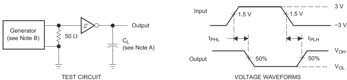
图 6-2. Driver Pulse Skew
