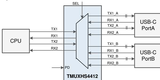
图 7-10. USB 4.0 / TBT 3.0 Demuxing
