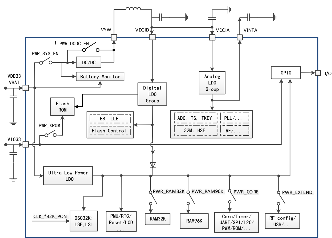
图 5-1 电源系统
