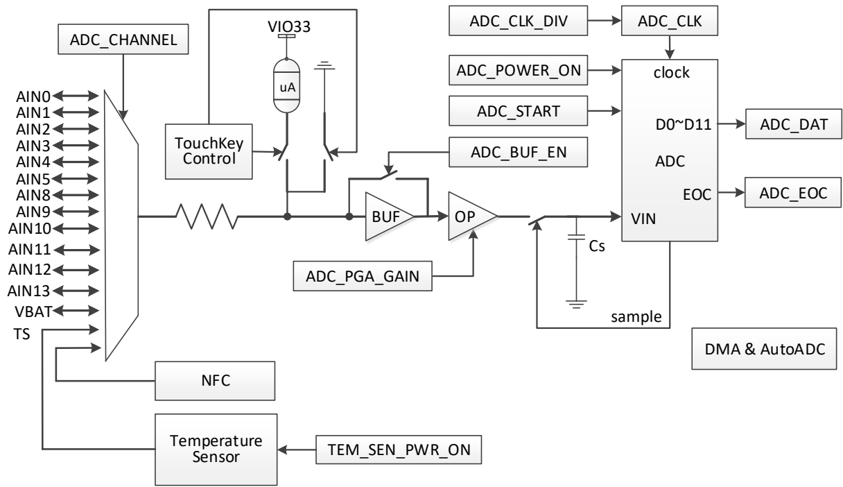
图 15-1 ADC 结构图
