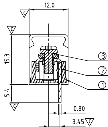
SECTION:P-P
