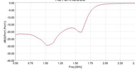
RETURNLOSS
