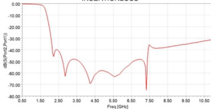
INSERTIONLOSS
