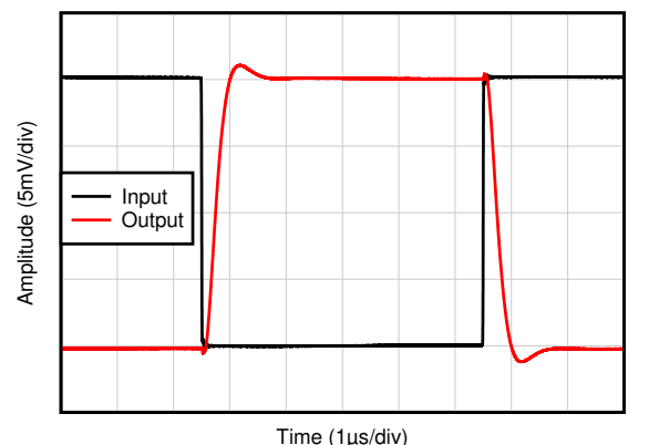
图 6-34. 负过载恢复
