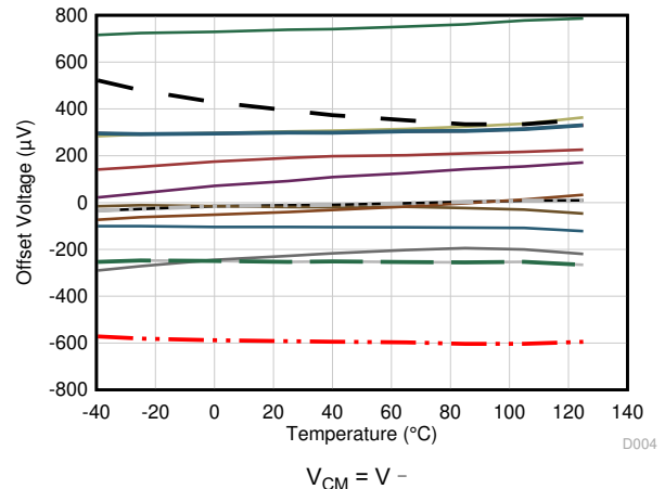
图 6-2. 失调电压漂移分配
