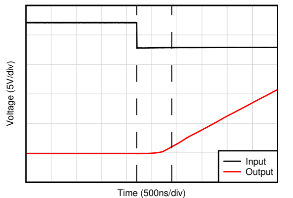
图 6-32. 无相位反转
