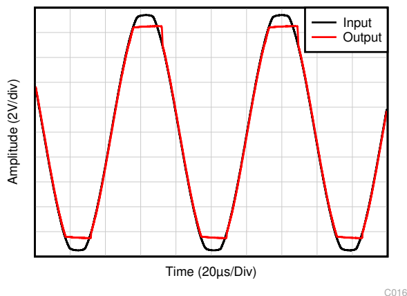
图 7-2. 无相位反转
