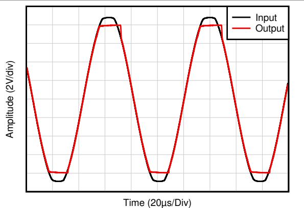
图 6-32. 无相位反转
