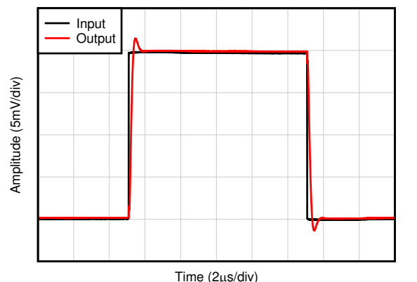
图 6-33. 正过载恢复
